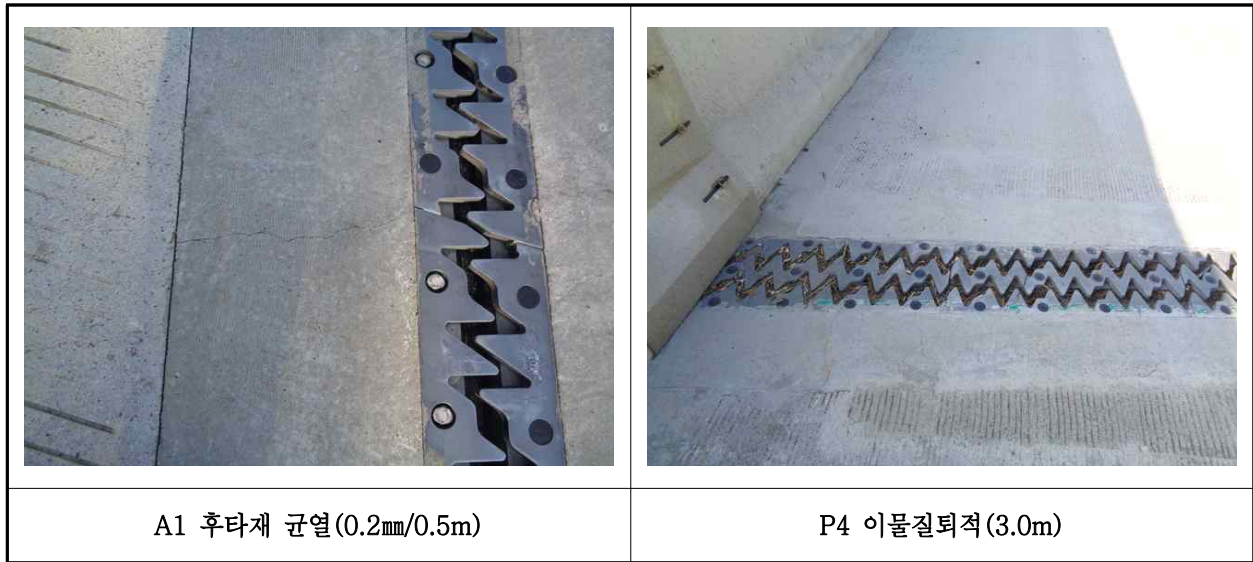
【사진 12.3.40】 신축이음장치 손상현황
