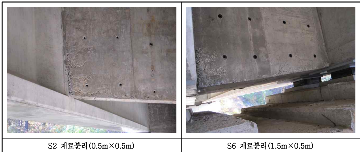
【사진 12.3.30】 가로보 손상현황
