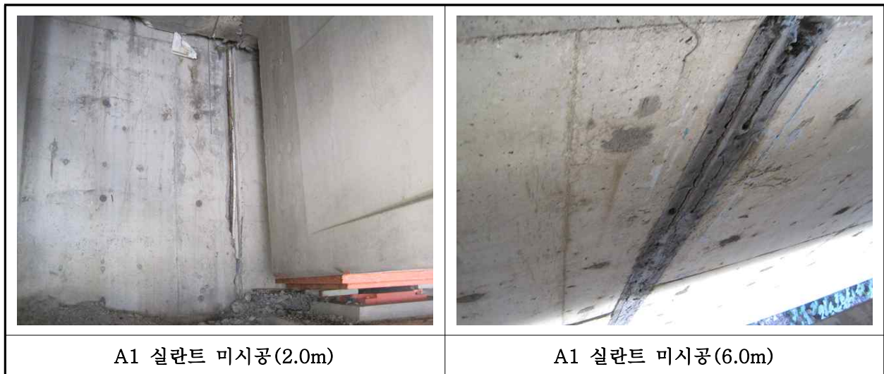
【사진 12.3.9】 교대 손상현황
