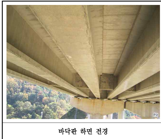
【사진 12.3.2】바닥판하면 전경
