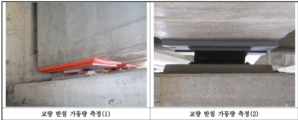
【사진 12.3.15】 교량받침 이동량 측정
